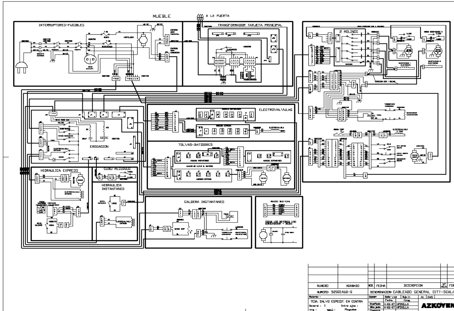
Referencia 52001460: Esquema del cableado general
